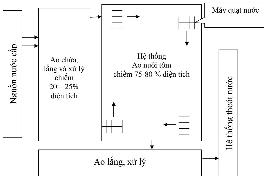
Sơ đồ mặt bằng hệ thống ao nuôi tôm nước lợ
